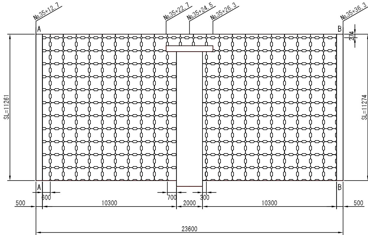
連節ブロック工展開図例 (No.35+24.5)
